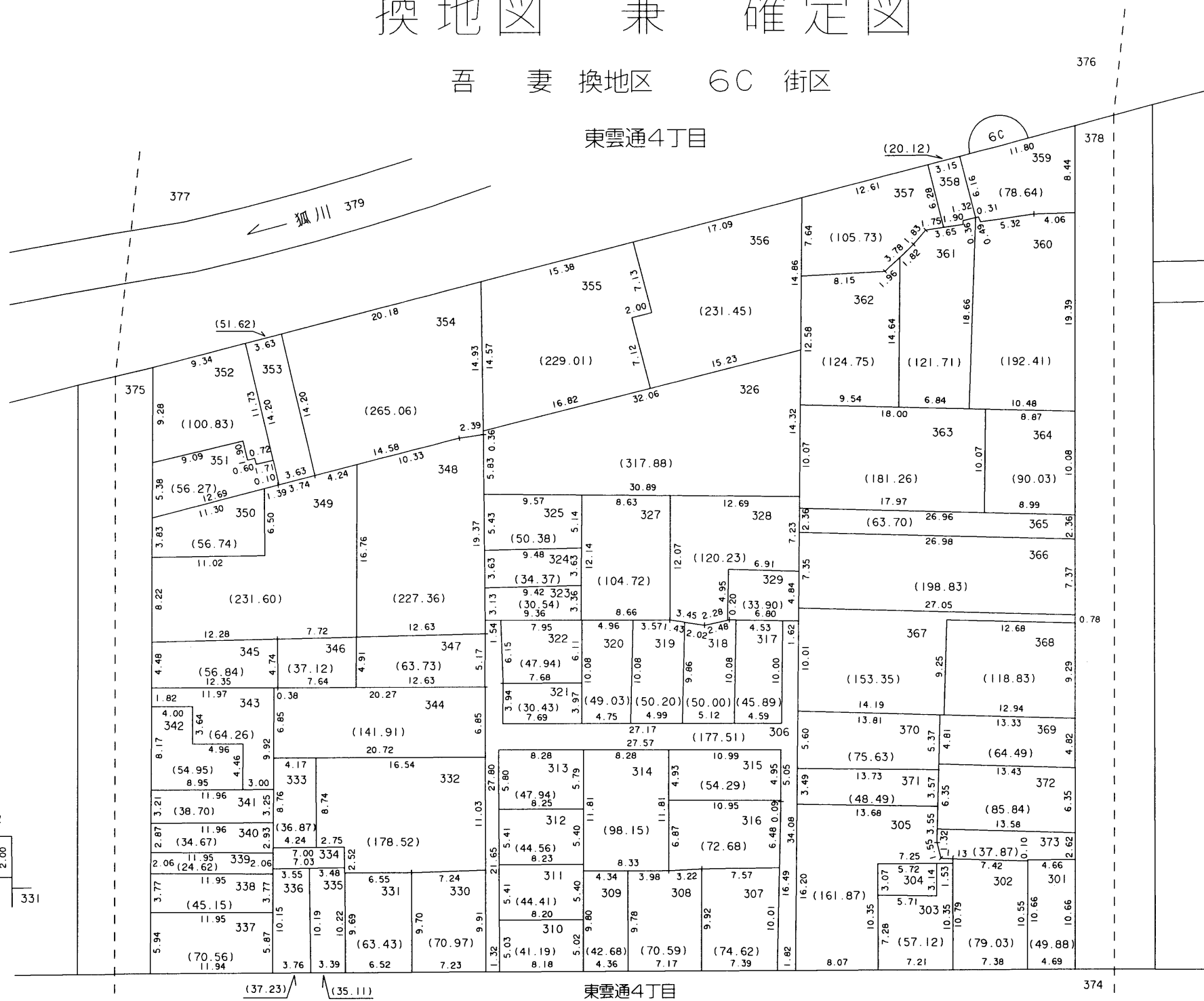
334 付近 略図
