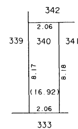
340 付近 略図
