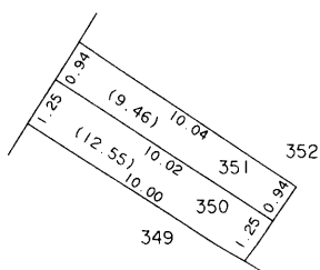
350 付近 略図
