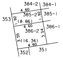
385-2 付近 略図
