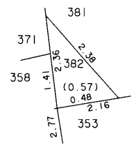
385-2 付近 略図
