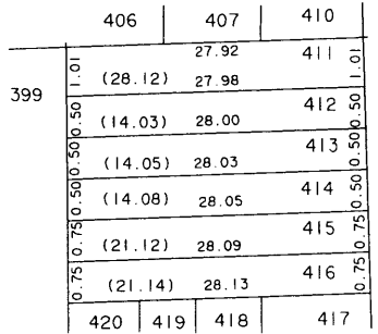
411 付近 略図
