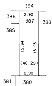
387 付近 略図
