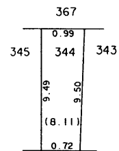
344 付近 略図
