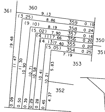
354 付近 略図
