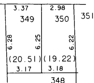
349 付近 略図
