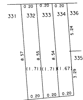
332 付近 略図
