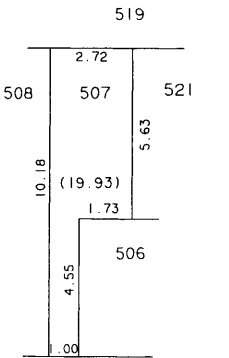
507 付近 略図
