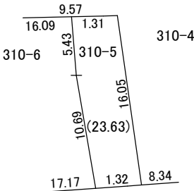
310-5 付近略図
