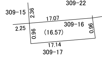
309-19 付近略図
