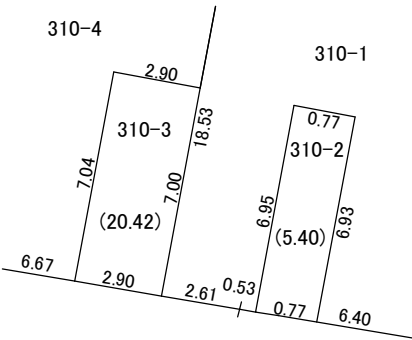
310-5 付近略図
