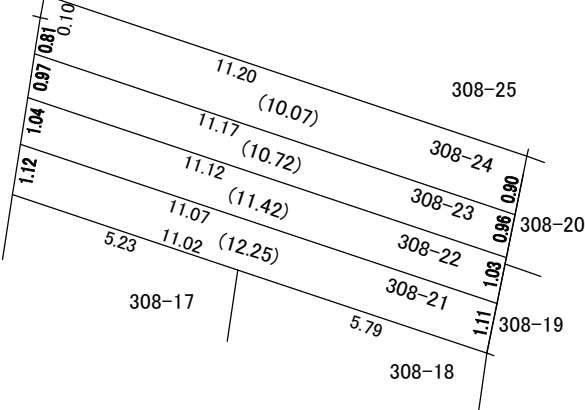
308-21 付近略図
