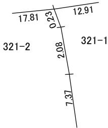
320-6 付近略図
