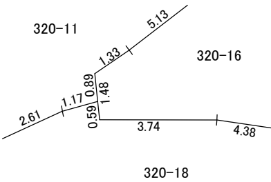
320-18 付近略図
