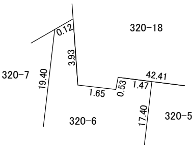
320-6 付近略図
