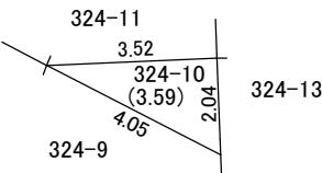
324-10 付近略図
