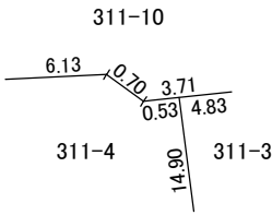
311-4 付近略図
