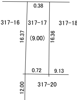
317-17 付近略図
