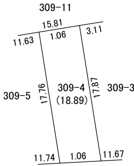
309-4 付近略図
