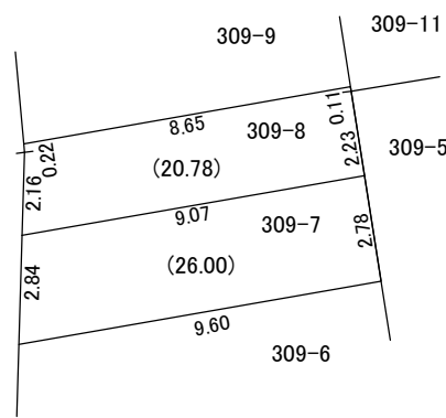
309-7 付近略図
