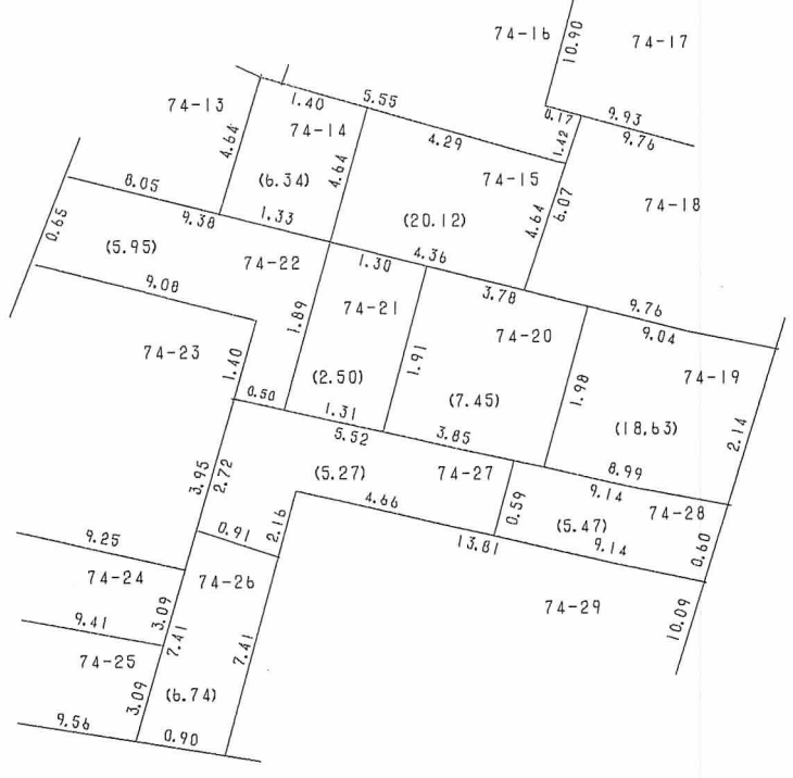
略図
