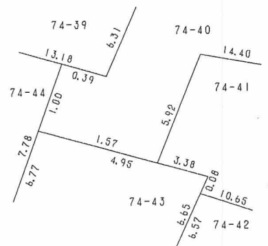
略図
