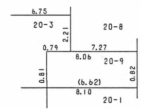
略図
