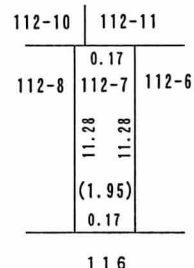
112-7 付近 略図
