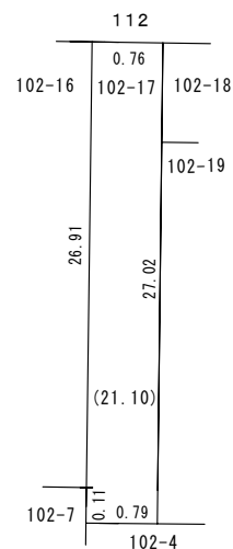
102-17 略図
